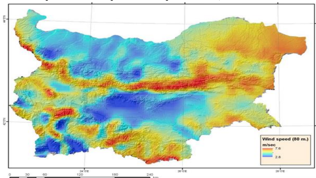
Карта 4. Теоретичен ветрови потенциал на височина 80 m
