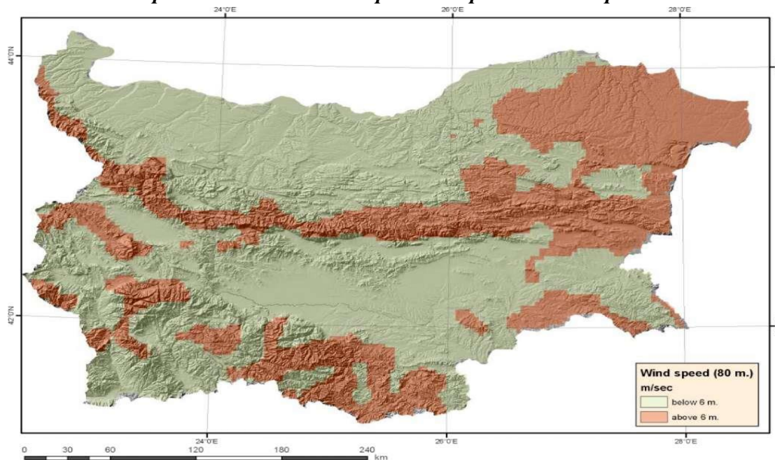
Карта 5. Годишна средна скорост на вятъра на 6 m/s.
